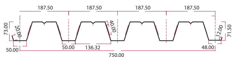
Σχήμα 3: Γεωμετρία του τραπεζοειδούς χαλυβδόφυλλου SYMDECK 73.
