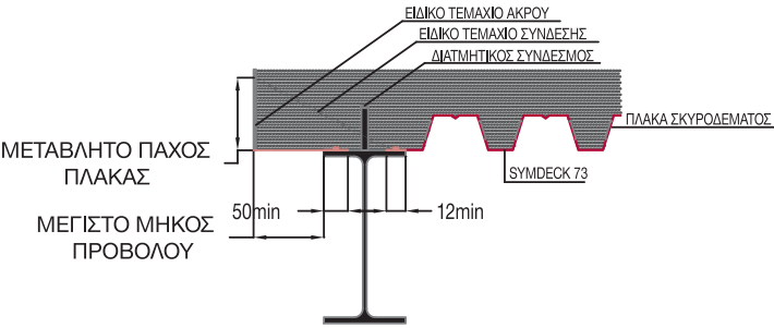
ΛΕΠΤΟΜΕΡΕΙΑ ΑΚΡΟΥ ΜΕ ΠΡΟΒΟΛΟ
